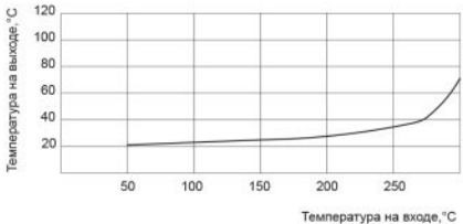
График для отвода-охладителя OC200-OX50
