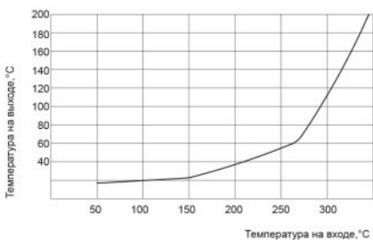
График для отвода-охладителя OC100-OX50
