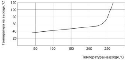
График для отвода-охладителя OC70-OX50
