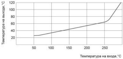
График для отвода-охладителя OC100-OX28
