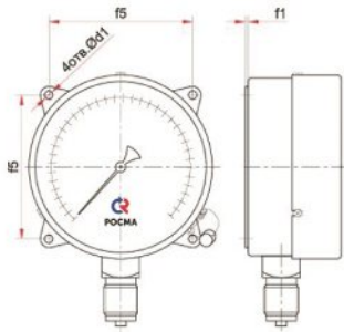
Радиальное присоединение с задним фланцем (Ø100, 150 мм)
