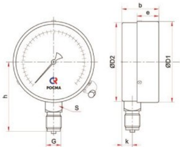
Радиальное присоединение (Ø100, 150 мм)
