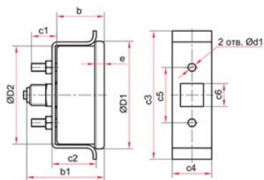
Осевое присоединение со скобой (Ø63 мм)
