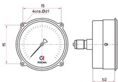
Осевое присоединение с передним фланцем (Ø100 мм)
