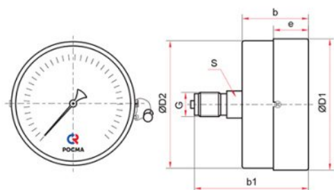
Осевое присоединение (Ø40, 50, 63, 100 мм)
