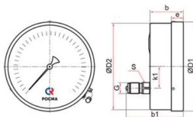
Эксцентрическое присоединение (Ø150, 160 мм)
