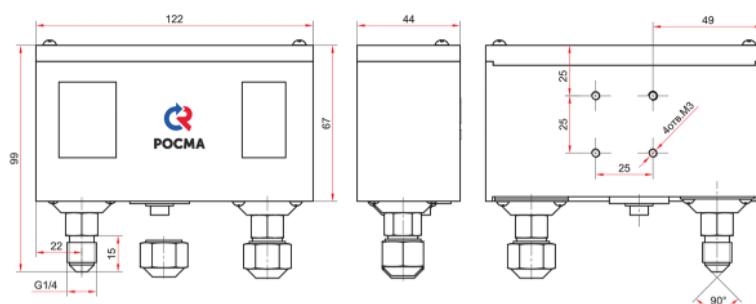
Реле давления РД-2Р двойное
