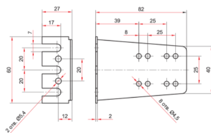
Кронштейн реле давления
