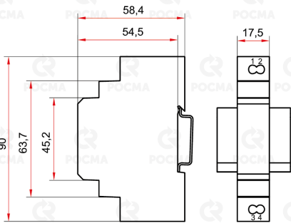
HDR-15-24
