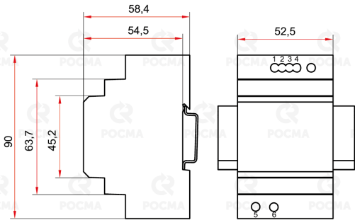
HDR-60-24
