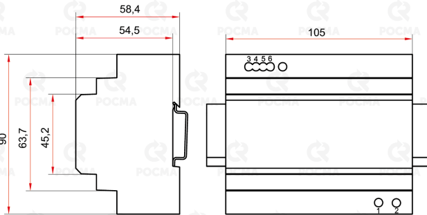
HDR-150-24
