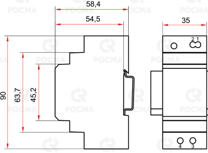
HDR-30-24
