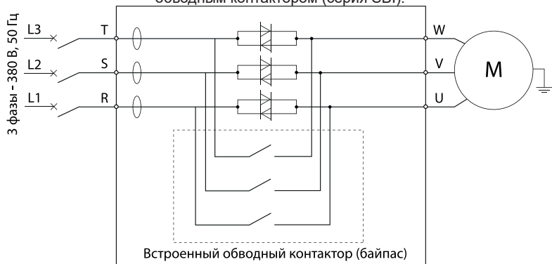
Схема подключения двигателя «в линию» для устройства плавного пуска с встроенным обводным контактором (серия SBI).
