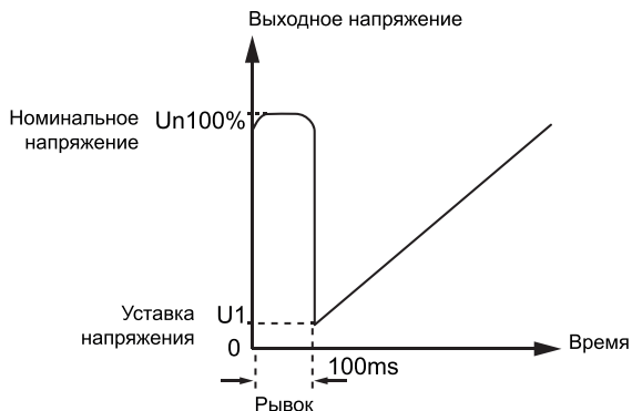
Запуск рывком + рампа по напряжению
