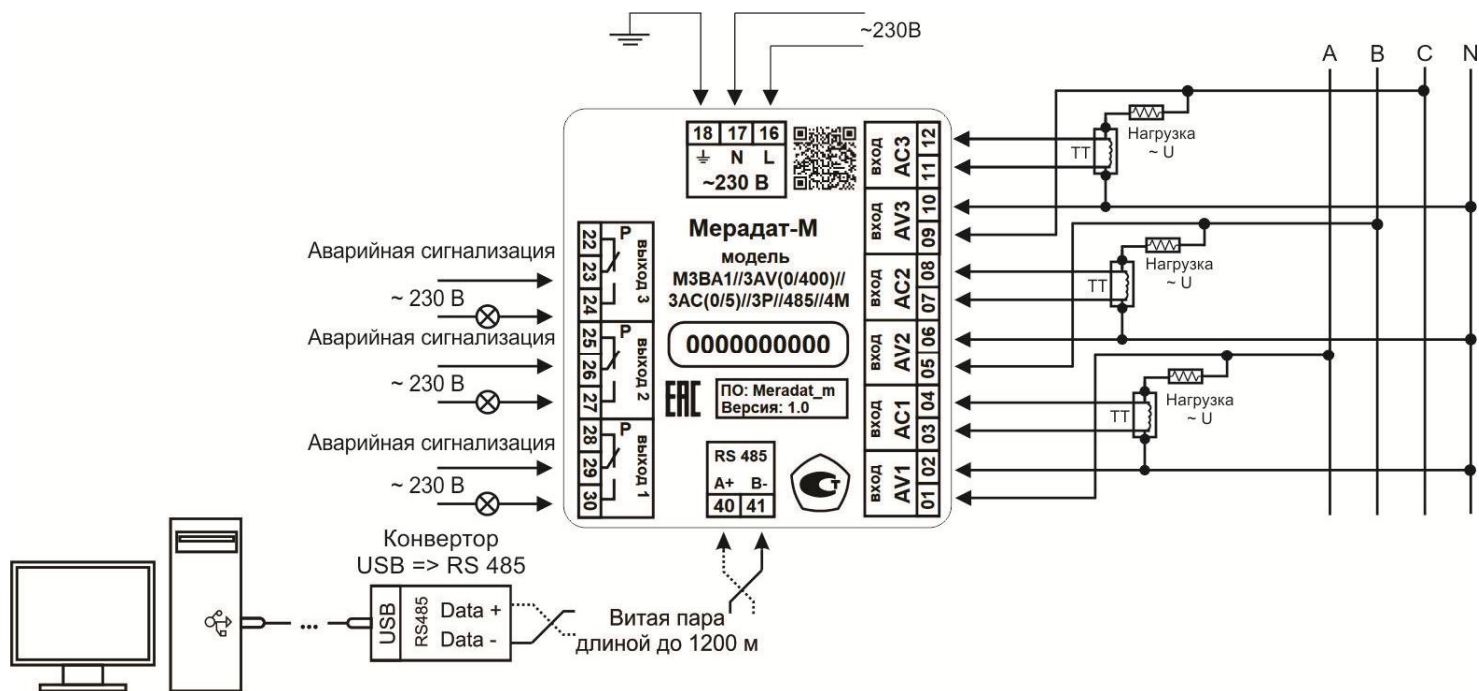
Рисунок 12 - Схема подключения МЗВ1//ЗАС(0/400)//...
